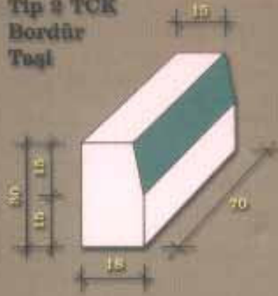
Kaldırım Bordür Taşı
